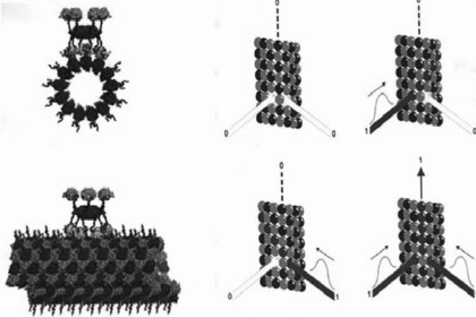
Anbindung des CaMKII an ein A-Gitter des Mikrotubulus
